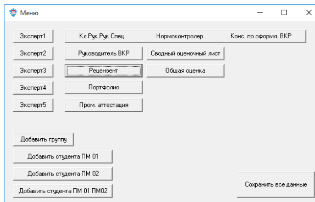
Рис. 12. Главное меню
