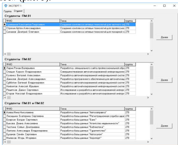
Рис. 5. Выбор студента
