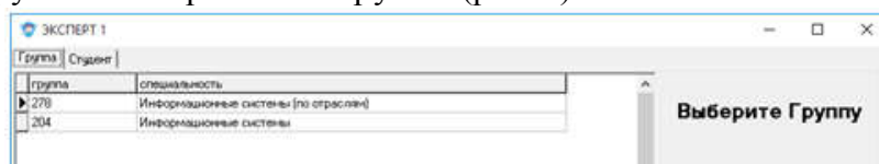
Рис. 4. Выбор Группы
